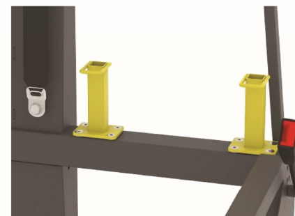
ISOFIX - Kindersitzbefestigung System ISOFIX child seats restraint system
